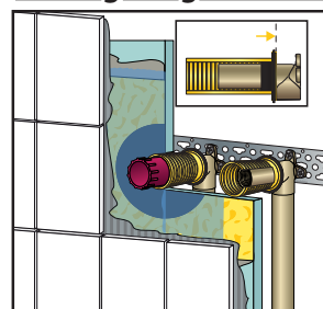
a: Für den Trockenbau
