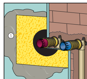
b: Für die konventionelle Wandmontage (Mauervariante)
